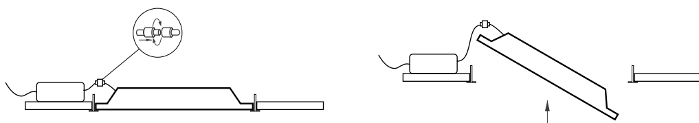
Рис. 2. Установка и подключение светильника
