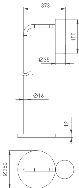
Рис. 1. Чертеж и габаритные размеры
