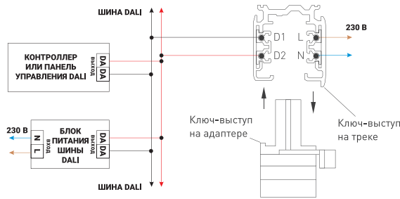
Рис. 2. Схема подключения светильников с управлением DALI
