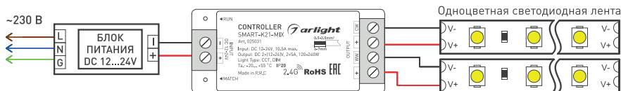
Рис. 2. Подключение одноцветной светодиодной ленты. Ленты управляются синхронно.
