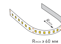
Рис. 4. Вертикальный радиус изгиба ленты
