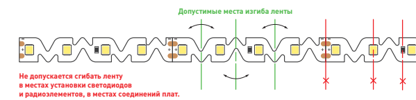
Рис. 5. Места сгиба ленты
