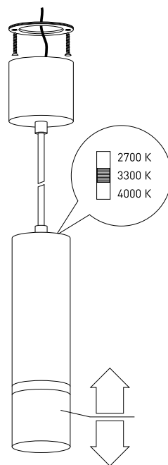
Рис. 2. Установка и подключение светильника
