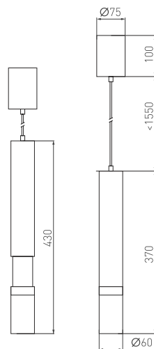
Рис. 1. Чертеж и габаритные размеры
